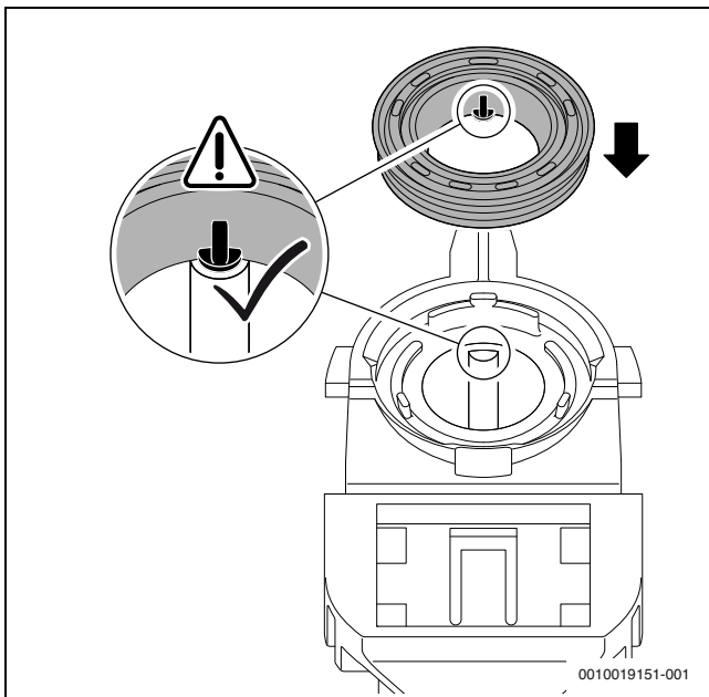
Fig. 60 Ajustarea garniturii noi pe sifonul pentru condensat
