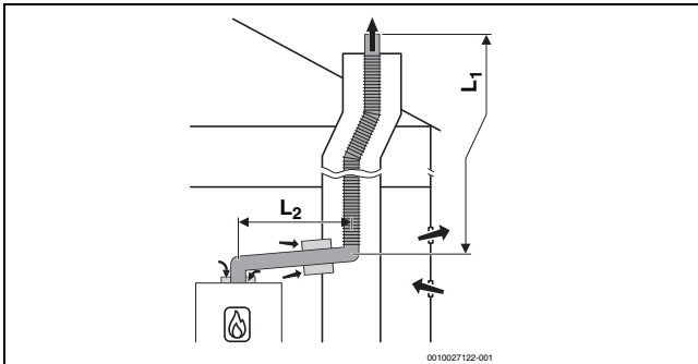
Fig. 19 Ghidarea flexibilă a gazelor arse în puț conform B 23p /B 53p cu alimentare cu aer dependentă de aerul din încăntă la nivelul aparatului și elementului de legătură concentric dintre încăperea centralei termice și puț
