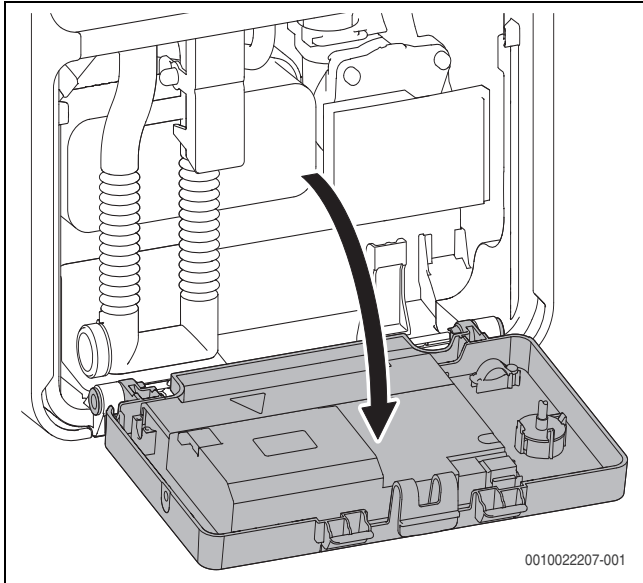
Fig. 33 Rabatarea echipamentului electronic în jos
