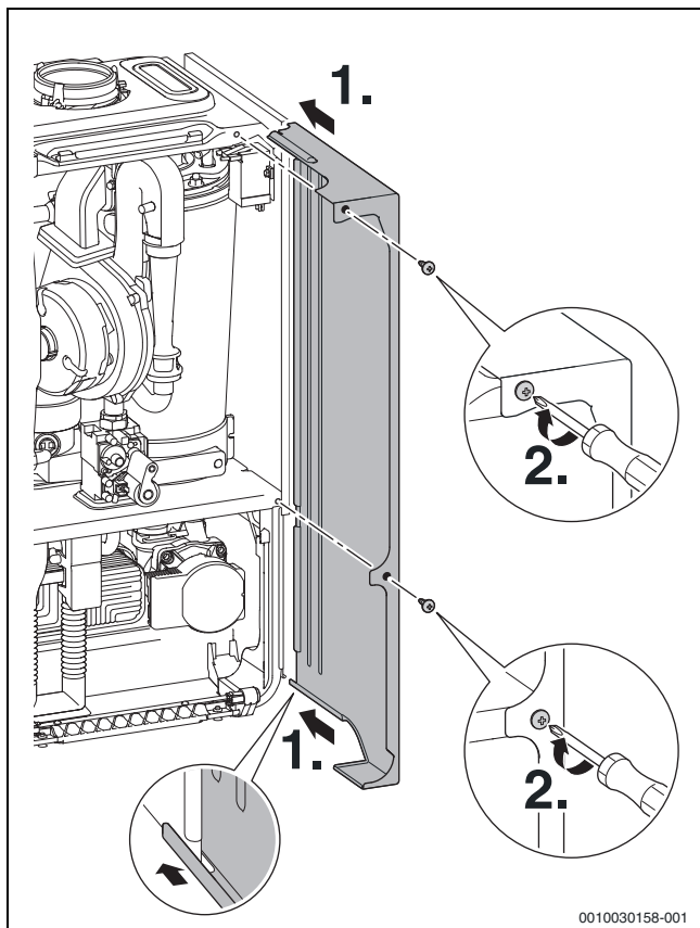
Fig. 75 Fixarea din nou a mantalei laterale
