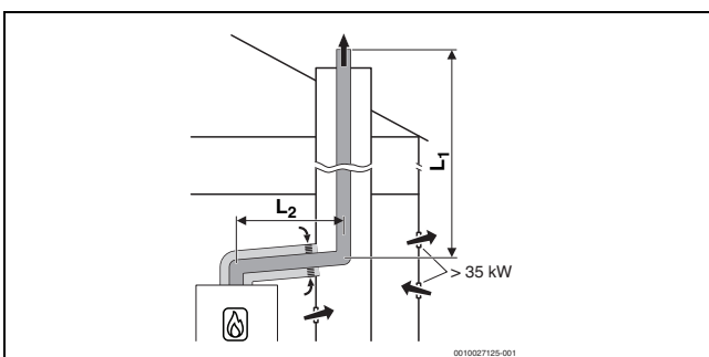
Fig. 20 Ghidarea rigidă a gazelor arse în puț conform B 33 cu alimentare cu aer dependentă de aerul din încăntă prin ghidarea concentrică a aerului/gazelor arse în încăperea centralei termice
