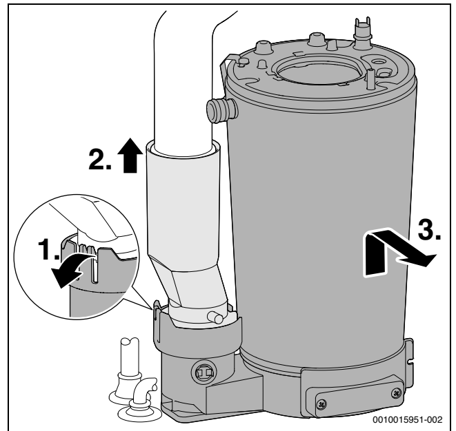
Fig. 72 Demontarea schimbatorului de căldură
