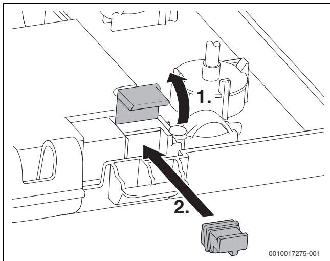
Fig. 74 Introduceți ștecăru de codare
