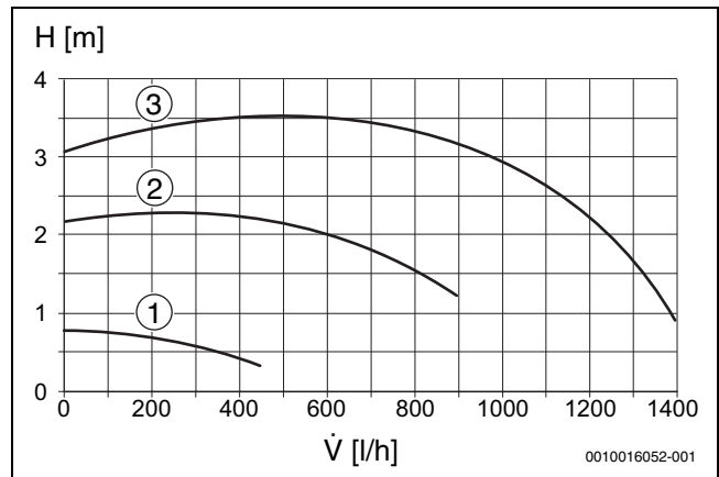
Fig. 41 Curba caracteristică a pompei pentru circuitul de încălzire (presiune proporțională)
