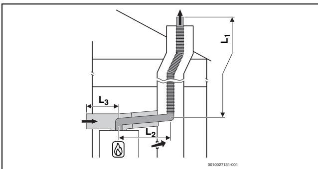
Fig. 13 Ghidarea flexibilă a gazelor arse în puț conform C 53x și ghidarea aerului/gazelor arse cu alimentare cu aer separată și evacuare concentrică a gazelor arse în încăperea centralei termice
