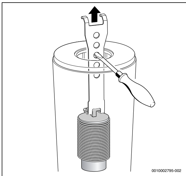
Fig. 53 Scoaterea corpului de întrepătrundere inferior
