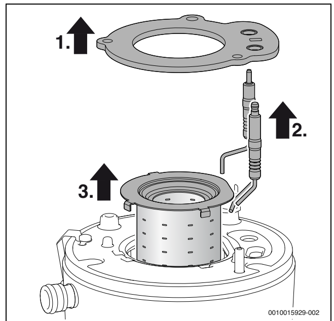
Fig. 51 Scoaterea arzătorului
