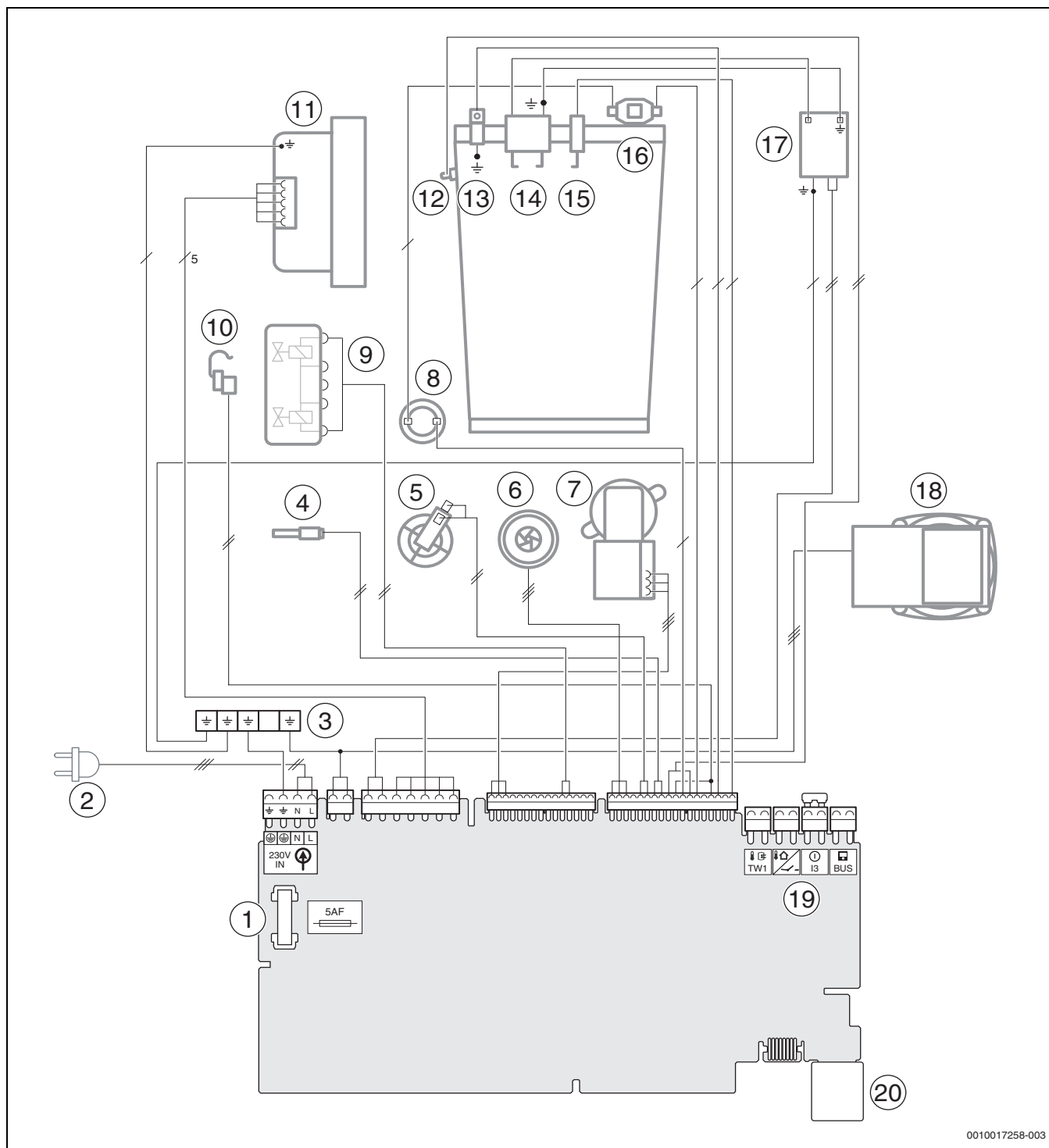
Fig. 78 Cablare electrică
