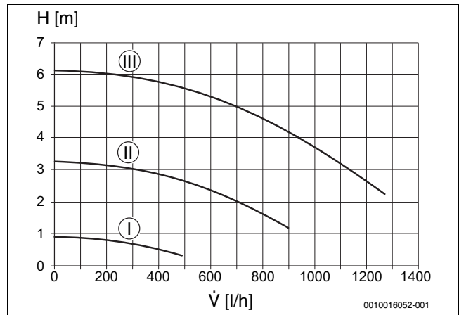
Fig. 39 Curba caracteristică a pompei pentru circuitul de încălzire (turație constantă)
