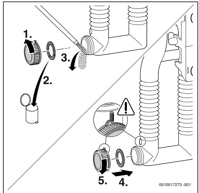
Fig. 58 Curățarea sifonului pentru condensat
