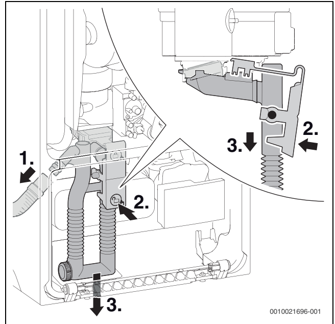
Fig. 57 Demontarea sifonului pentru condensat
