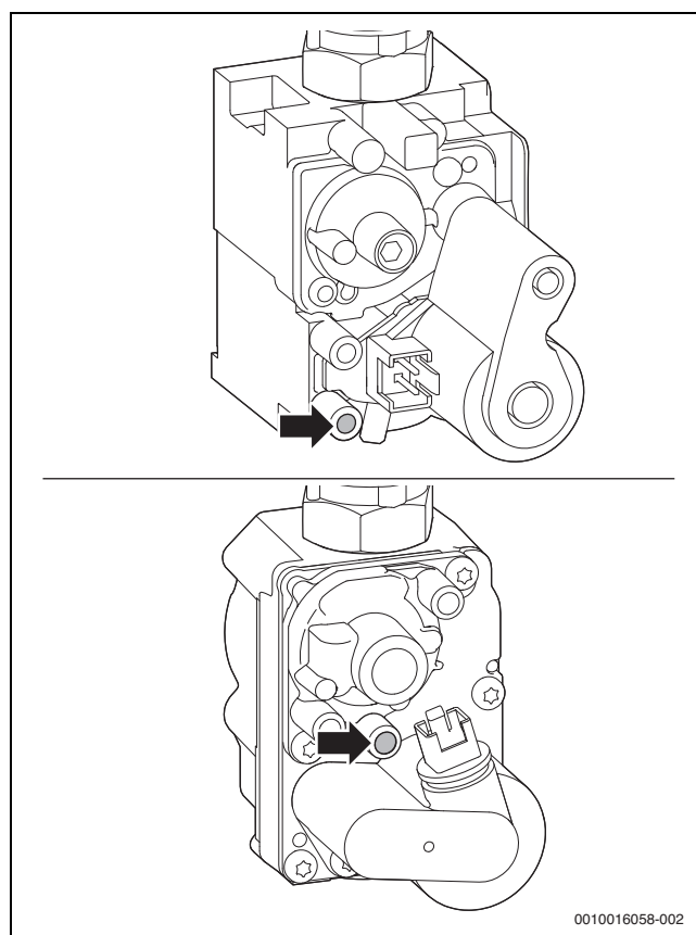
Fig. 45 Orificiul de măsurare pentru presiunea de racordare a gazului
