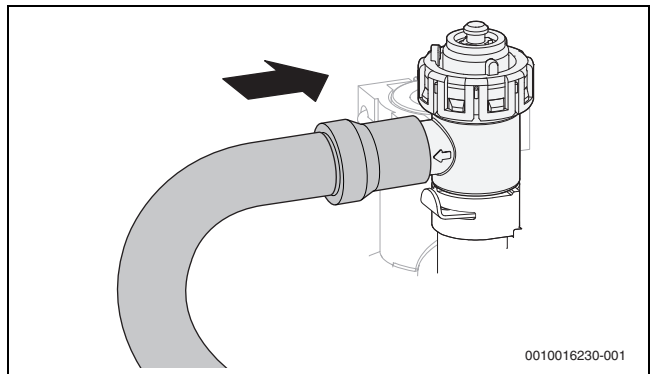
Fig. 29 Montarea furtunului la supapa de siguranță
