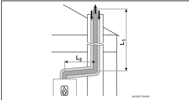
Fig. 8 Ghidarea concentrică a aerului/gazelor arse în puț conform C 33x
