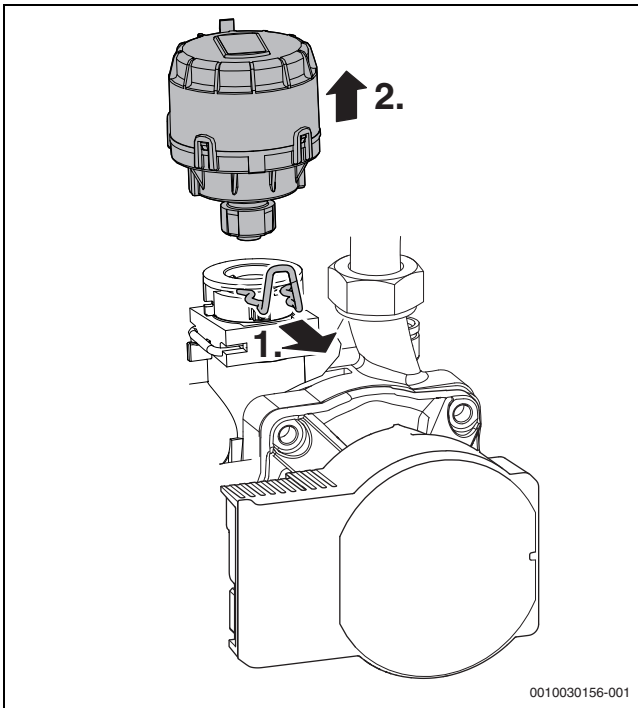
Fig. 70 Demontarea motorului vanei cu 3 căi
