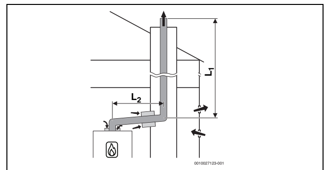
Fig. 18 Ghidarea rigidă a gazelor arse în puț conform B 23p /B 53p cu alimentare cu aer dependentă de aerul din încăpărea aparatului și elementului de legătură concentric dintre încăpărea centralei termice și puț
