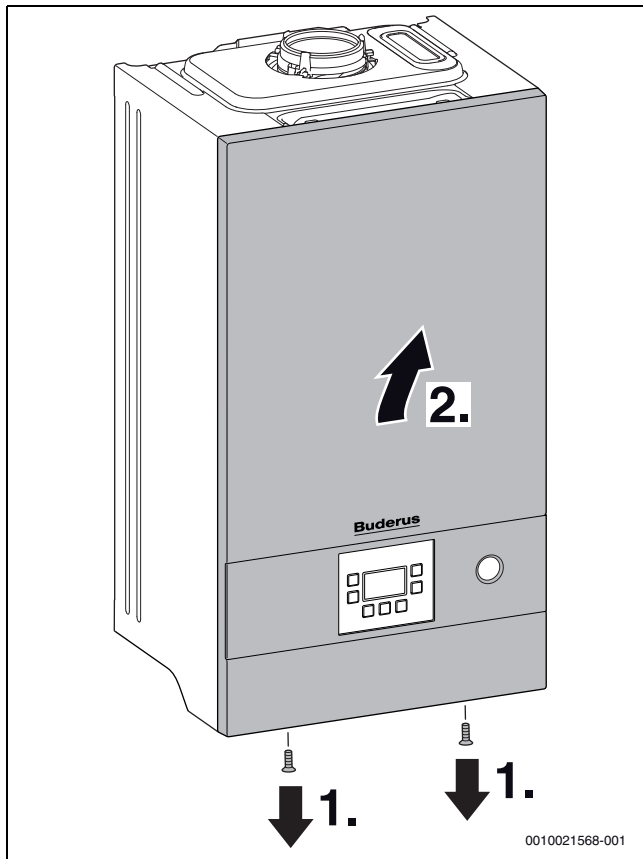
Fig. 28 Scoaterea mantalei frontale
