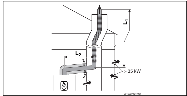
Fig. 21 Ghidarea flexibilă a gazelor arse în puț conform B 33 cu alimentare cu aer dependentă de aerul din încăntă prin ghidarea concentrică a aerului/gazelor arse în încăperea centralei termice
