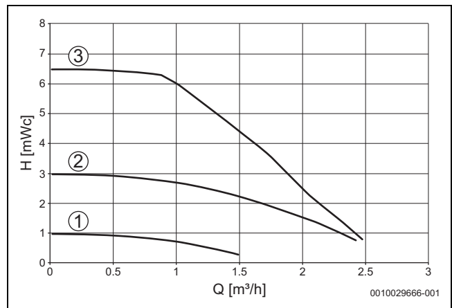
Fig. 40 Curbă caracteristică a pompei pentru circuitul de încălzire (presiune constantă)
