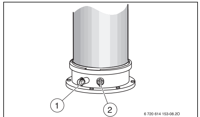
Fig. 46 Orificiul de măsurare a gazelor arse și orificiul de măsurare a aerului de ardere
