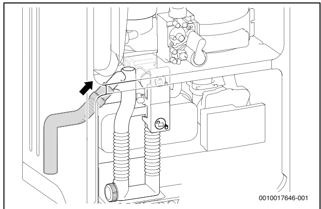
Fig. 30 Montarea furtunului la sifonul pentru condensat
