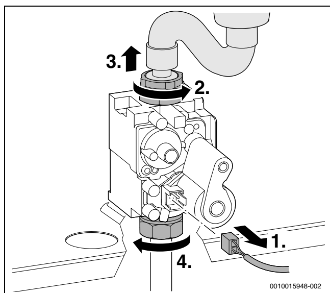
Fig. 66 Scoaterea ștecărului și desfacerea piulițelor orbe
