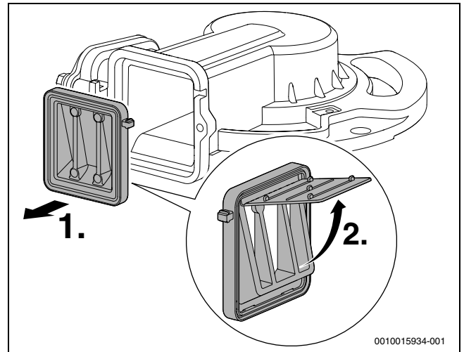
Fig. 50 Clapeta de sens din sistemul de amestecare
