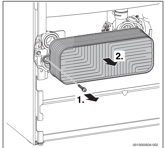
Fig. 65 Demontarea schimbătorului de căldură în plăci
