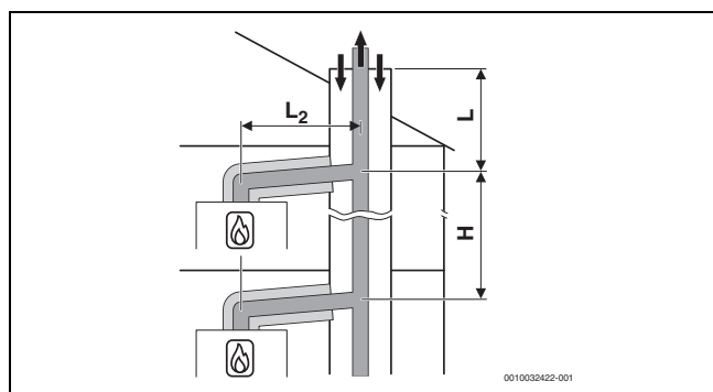
Fig. 24 Acoperire multiplă conform C (14)3x cu ghidarea colectivă rigidă a gazelor arse și ghidarea concentrică a aerului/gazelor arse în încăperea centralei termice
